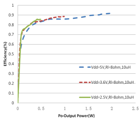
效率 vs. 输出电压(8ohm)
