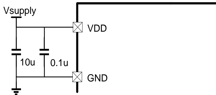
Fig.26. 电源去耦
