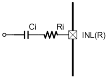
Fig.24. MT6868: 单端输入
