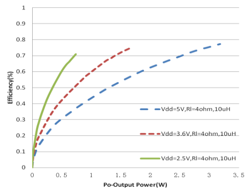
效率 vs. 输出电压(ABmode)
