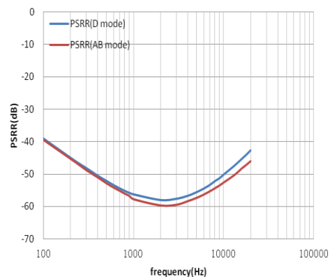
PSRR vs. 频率
