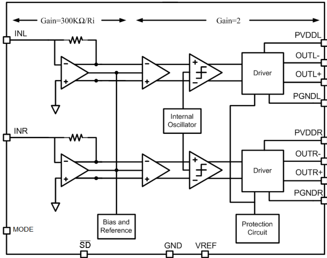
芯片内部框图
