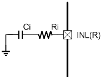
Fig.25. MT6868: 不用通道输入端的连接
